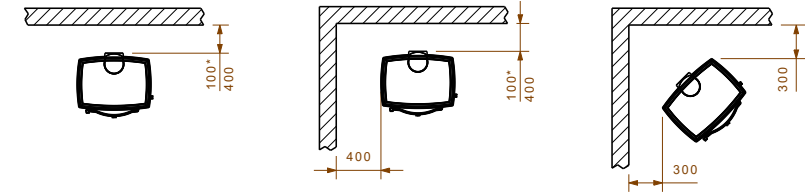
Avstand til brennbart materiale
