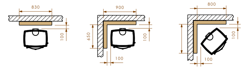
Utenpåliggende brannmur
