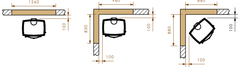
Utenpåliggende brannmur
