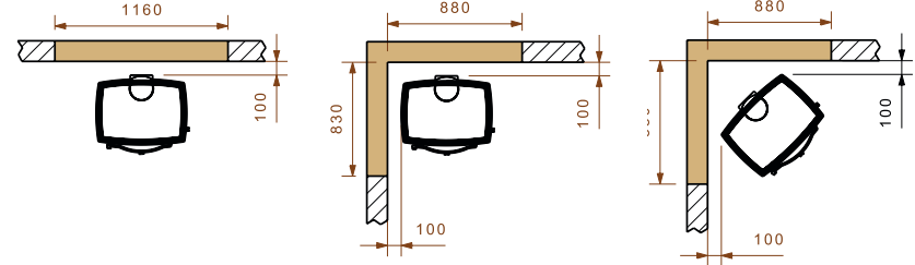
Utenpåliggende brannmur
