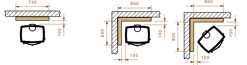
Utenpåliggende brannmur
