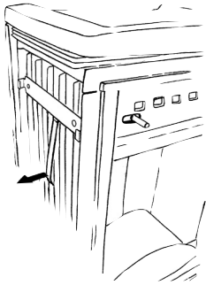
Fig. 6 Bøy ut fjæren før monteringen av sideplater
