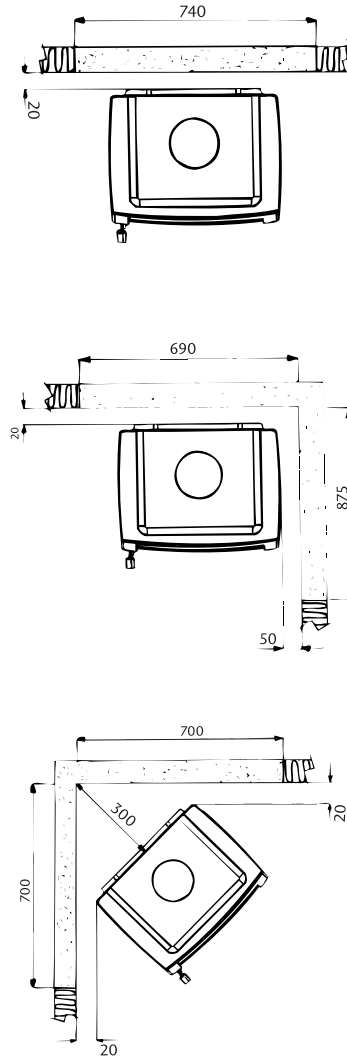
Innfelt brannmur. Brannmurens høyde over ildstedet skal være min. 300 mm
