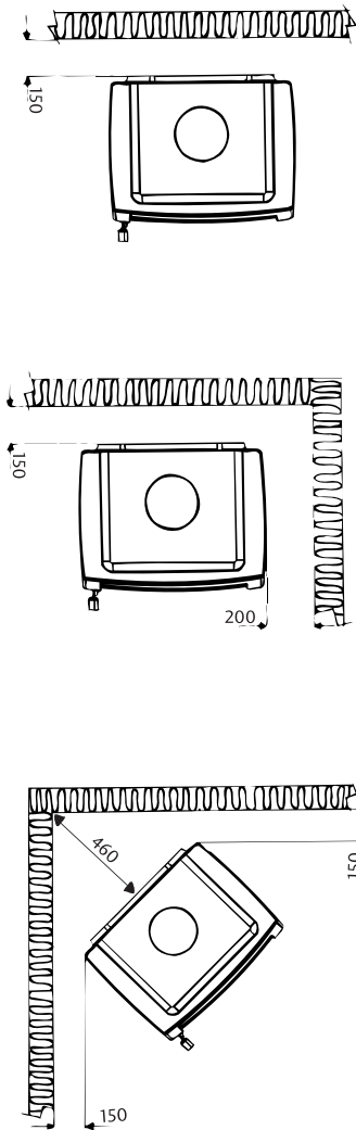
Vegg av brennbart materiale
