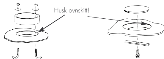
Fig. 4 Montering blindlokk (angrelokk)
