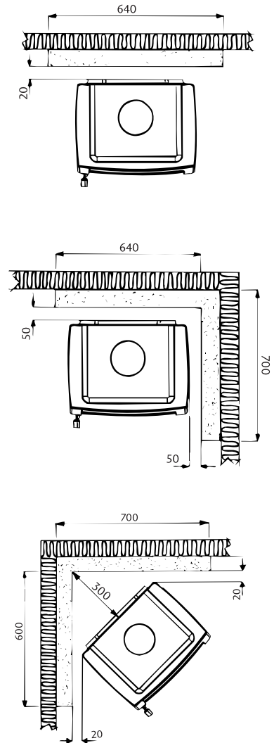
Utenpåliggende brannmur. Brannmurens høyde over ildstedet skal være min. 200 mm
