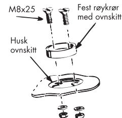
Fig. 3. Montering av røykuttak
