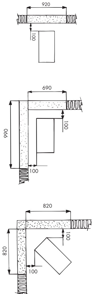
Min. mål utpåliggende brannmur
