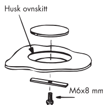
Fig. 4 . Montering blindlokk
