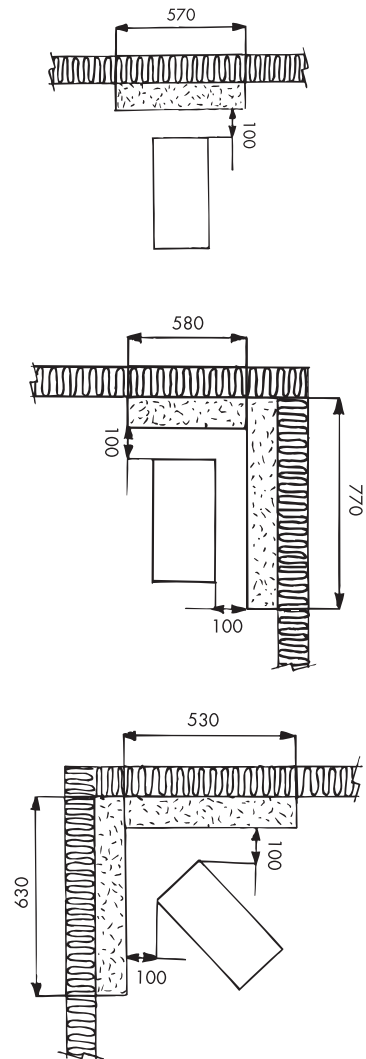
Min. mål innfelt brannmur
