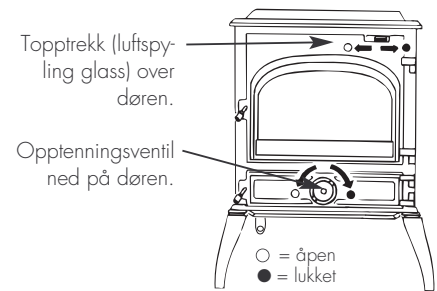
Fig. 10 Betjening trekkregulering
