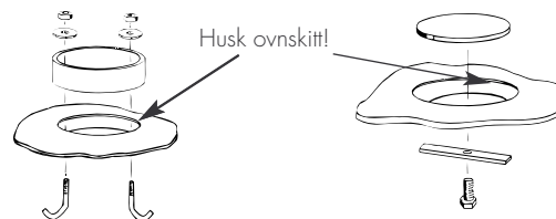
Fig. 3 Montering røykstuss
