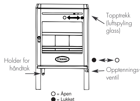
Fig. 7 Betjening trekkregulering
