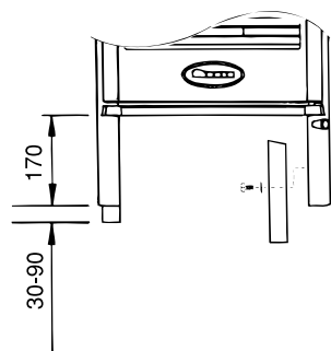
Fig. 5 Montering av bein og høydejustering (tilleggsutstyr)
