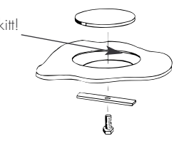
Fig. 4 Montering blindløkk (angreløkk)
