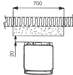
Utenpåliggende brannmur. Brannmurens høyde over ildstedet skal være min. 200 mm
