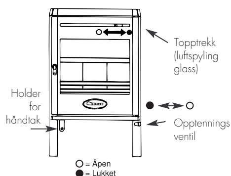
Fig. 7 Betjening trekkregulering
