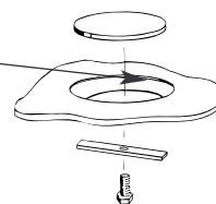
Fig. 4 Montering blindlokk (angreløkk)
