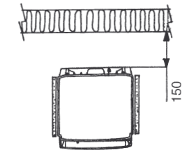
Avstand til vegg av brennbart materiale med marmor-sideplater på ovnen
