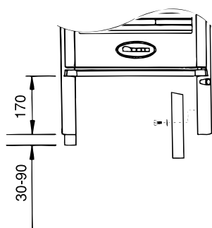
Fig. 5 Montering av ben og høydejustering (tilleggsutstyr)
