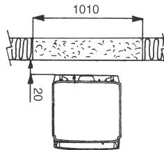
Innfelt brannmur. Brannmurens høyde over ildstedet skal være min. 300 mm
