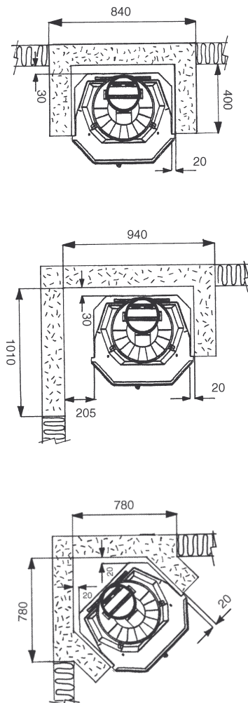
Min. mål innfelt brannmur
