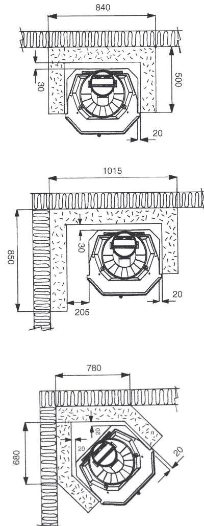
Min. mål utpåliggende brannmur
