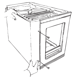
Fig. 2 Montering bakere varmeskjold med sideglass. Varmeskjoldene på sidene skal monteres når sideglass skal monteres ikke benyttes.
