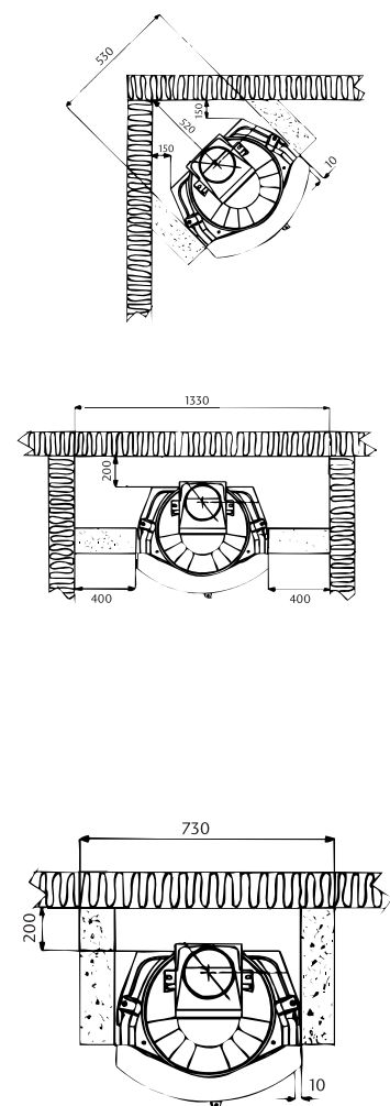
Min. mål mot brennbart materiale
