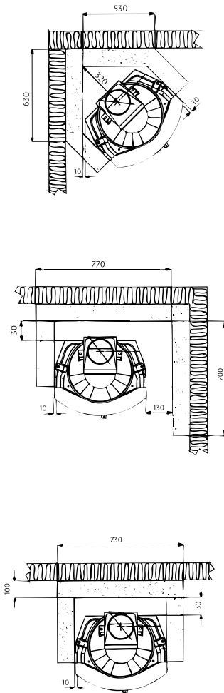
Min. mål utpåliggende brannmurmål
