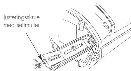
Fig. 4 Montering av bein
